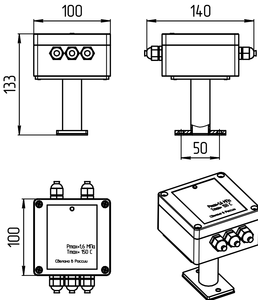
Рис6. Измерительный модуль М021
