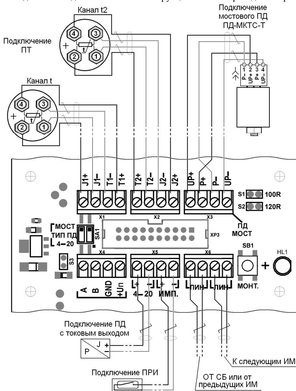
Рис11. Схема монтажа на плате подключений ИМ с типом конструкции И5 и К5
