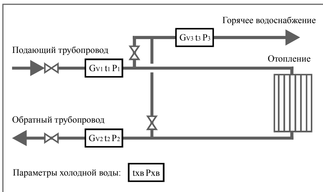
Рис25. Пример установки ИМ для узла учета с системами отопления и ГВС
